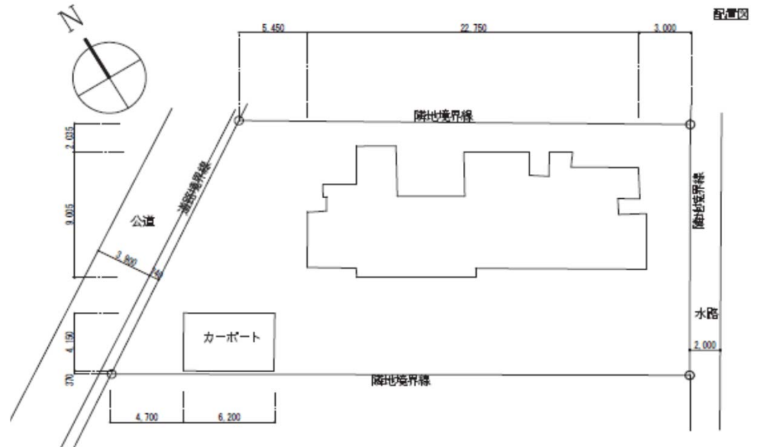
配置図
